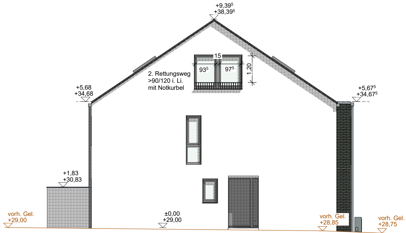
Ansicht Süd
